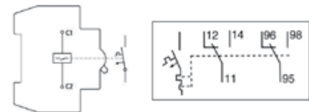
Schematic display of the shunt trip release Bobina de apertura representación esquemática
