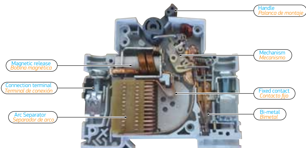
Main parts composing an miniature circuit breaker Las piezas principales que forman un fusible automático.
